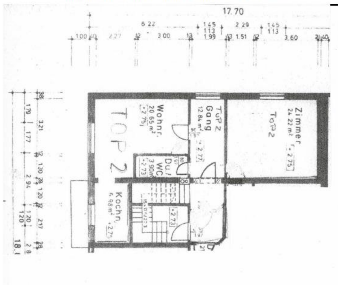
Abbildung 1: Grundriss Top 2, ca. 68,5 m 2
